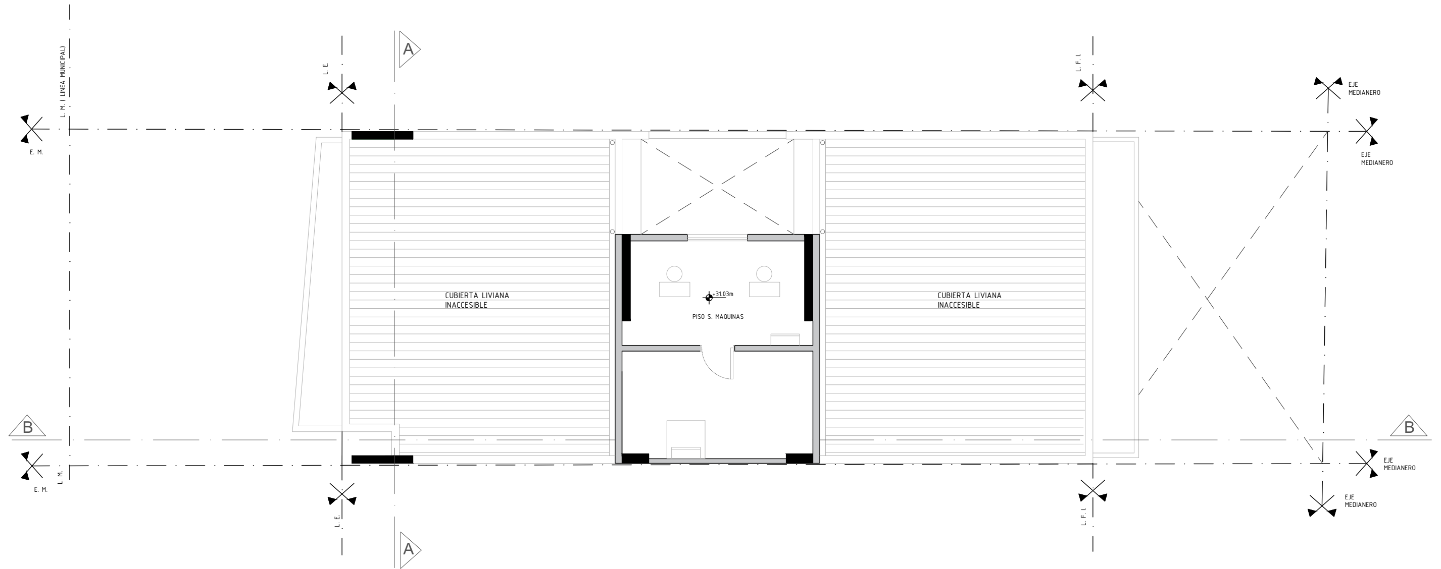
PLANTA CUBIERTA Y SALA DE MAQ.
