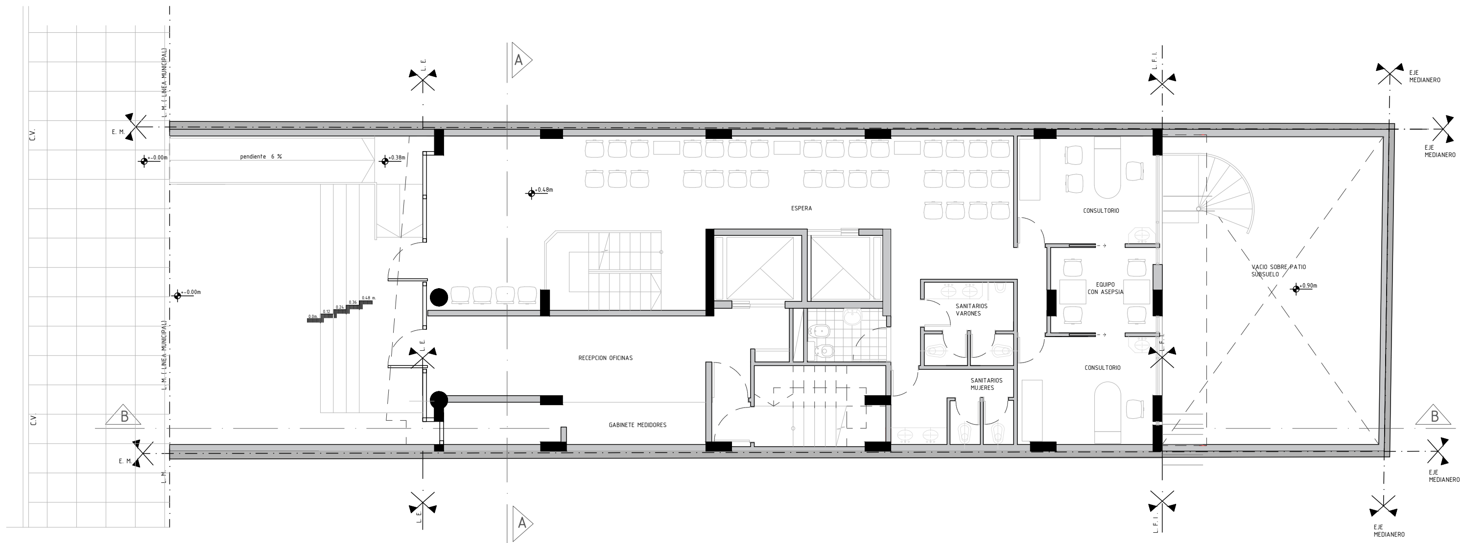
PLANTA BAJA
